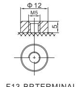
F13-BP TERMINAL
